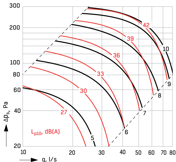
Diagram 2. a) Frånluftsfläkt, inställning potentiometer (V). b) Ljud till kök, L_{p10A} , från aggregat (båda fläktar körs) med stängt forceringsspjäll i spiskåpan. c) Filter (M5) ISO Coarse 85%. d) Om RDKS byggs in mellan två köksskåp tillsammans med frontlucka, så sjunker ljudnivån till omgivningen med 1 - 2 dB.
